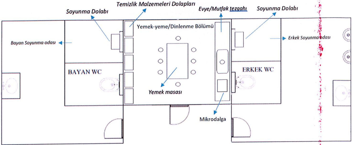
Şekil 3.2. Alsancak iskelesinde yapılacak iyileştirme çalışmaları kapsamında yapılacak Erkek, Bayan WC değişiklikleri ve Yemek yeme dinlenme alanı oluşturulmasını gösterir yeni yerleşim planı
